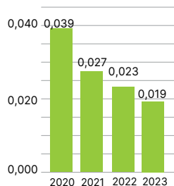
Residus Biològic/activitat
